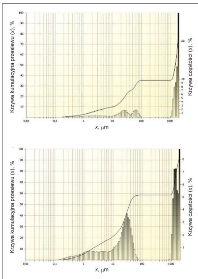
Rys. 5. Specyficzne rozkłady cząstek konkrecji rozdrobnionych w młynie hydrostrumieniowym przy ciśnieniu strugi wodnej 200 MPa
