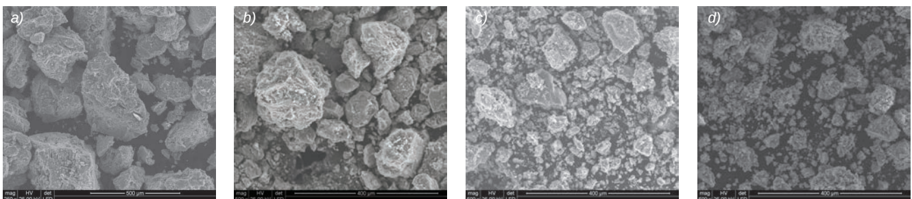
Rys. 3. Przykładowe obrazy SEM kongrecji polimetalicznych rozdrobnionych w młynie hydrostrumieniowym przy ciśnieniu strugi wodnej: a) 70 MPa, b) 100 MPa, c) 150 MPa, d) 200 MPa
