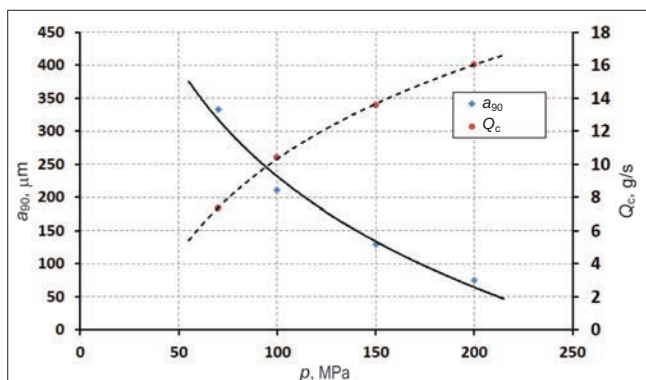
Rys. 4. Wpływ ciśnienia strugi wodnej na wielkość cząstek ( a_{90} ) rozdrobnionych konkrecji i wydajność ( Q_c ) procesu ich hydrostrumieniowego mielenia
