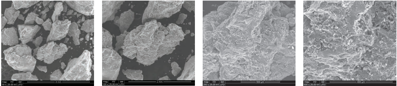
Rys. 1. Przykładowe obrazy SEM cząstek kongrecji polimetalicznych (z widokiem rozwinięcia ich powierzchni) rozdrobnionych w kruszarce szczękowej
