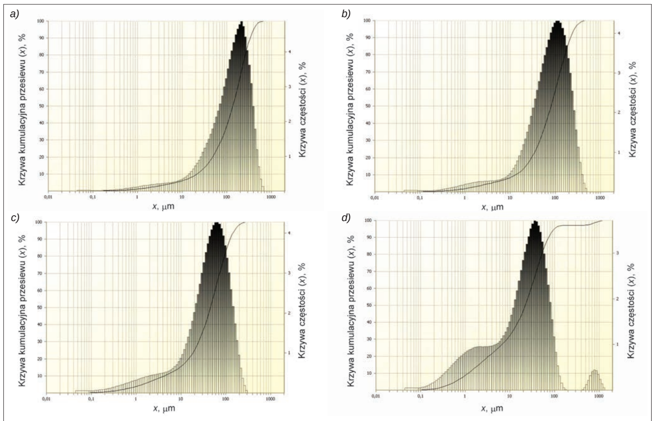
Rys. 2. Przykładowe rozkłady cząstek kongrecji polimetalicznych rozdrobnionych w młynie hydrostrumieniowym przy ciśnieniu strugi wodnej: a) 70 MPa, b) 100 MPa, c) 150 MPa, d) 200 MPa
