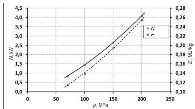
Rys. 6. Wpływ ciśnienia strugi wodnej na jej moc ( N ) i energię jednostkową ( E ) hydrostrumieniowego rozdrabniania konkrecji
